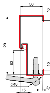
OCELOVÁ ZÁRUBEŇ
