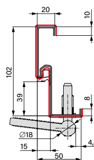
ROHOVÁ OCELOVÁ ZÁRUBEŇ
