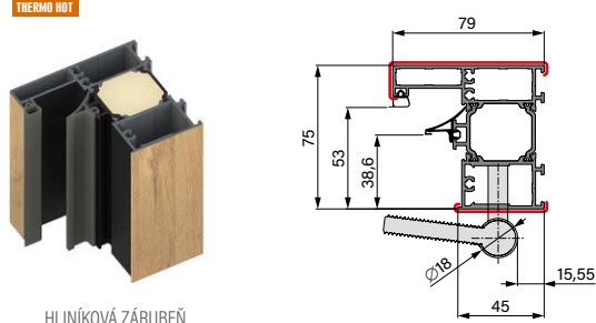
HLINÍKOVÁ ZÁRUBEŇ
