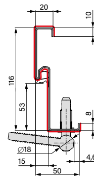
ROHOVÁ OCELOVÁ ZÁRUBEŇ
