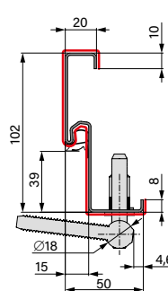
ROHOVÁ OCELOVÁ ZÁRUBŇA
