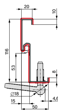
ROHOVÁ OCELOVÁ ZÁRUBŇA
