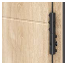
3D nastaviteľný pánt v čiernej farbe s dodatočnou ochrannou krytkou
