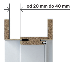
ZÁRUBŇA SO ŠIROKÝM PEROM príplatková možnosť
