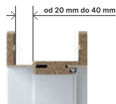
ZÁRUBŇA SO ŠÍROKÝM PEROM príplatková možnosť
