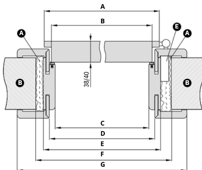
SCHÉMA NASTAVITELNEJ ZÁRUBNE
